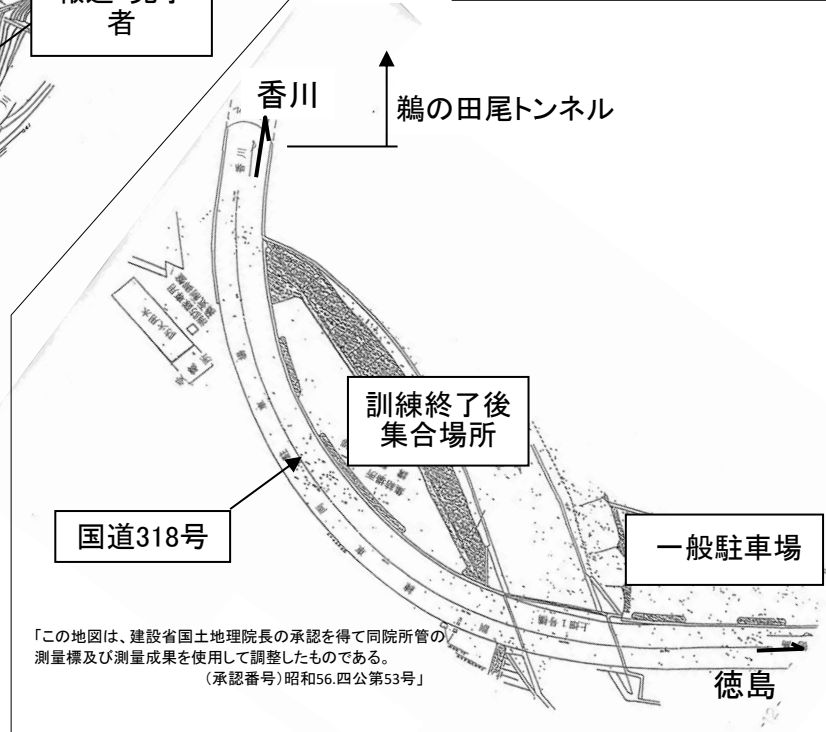
【図3】徳島県側坑口平面図
