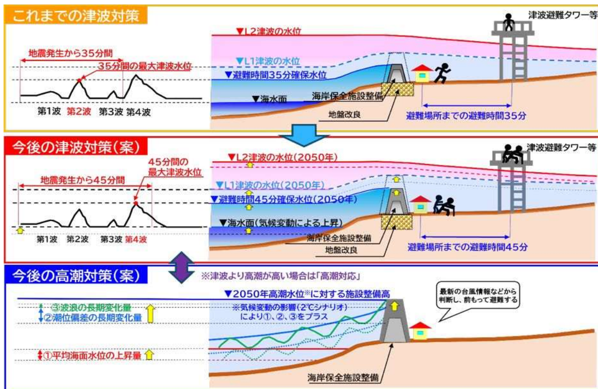
今後の海岸保全施設整備のイメージ
