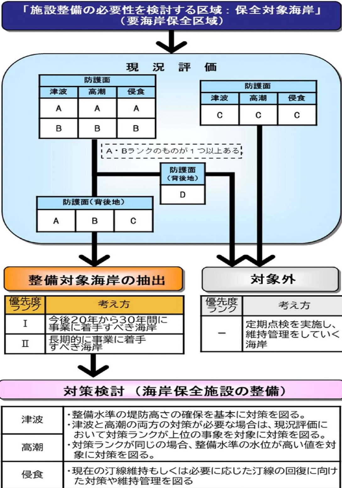
整備対象海岸の抽出・整備優先度の決定・対策検討のフロー
