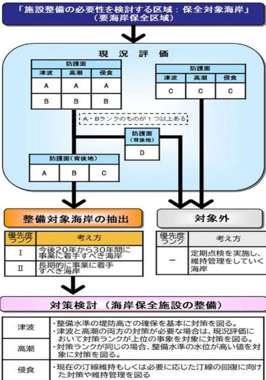
整備対象海岸の抽出・整備優先度・対策検討のフロー
