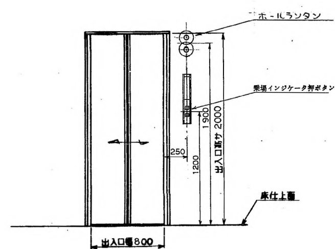
正面図 (1/20)
