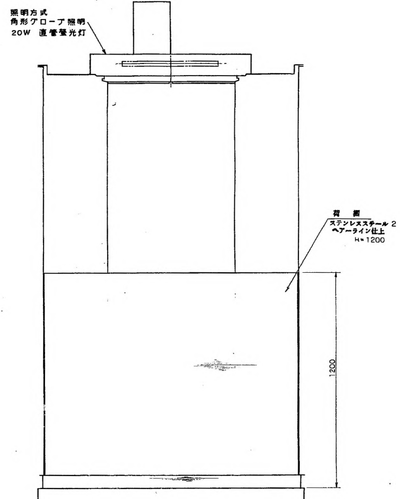
背面図
