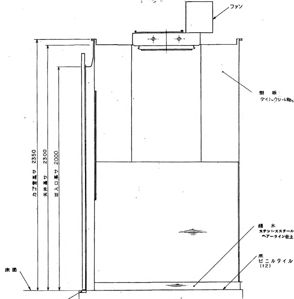
側面図
