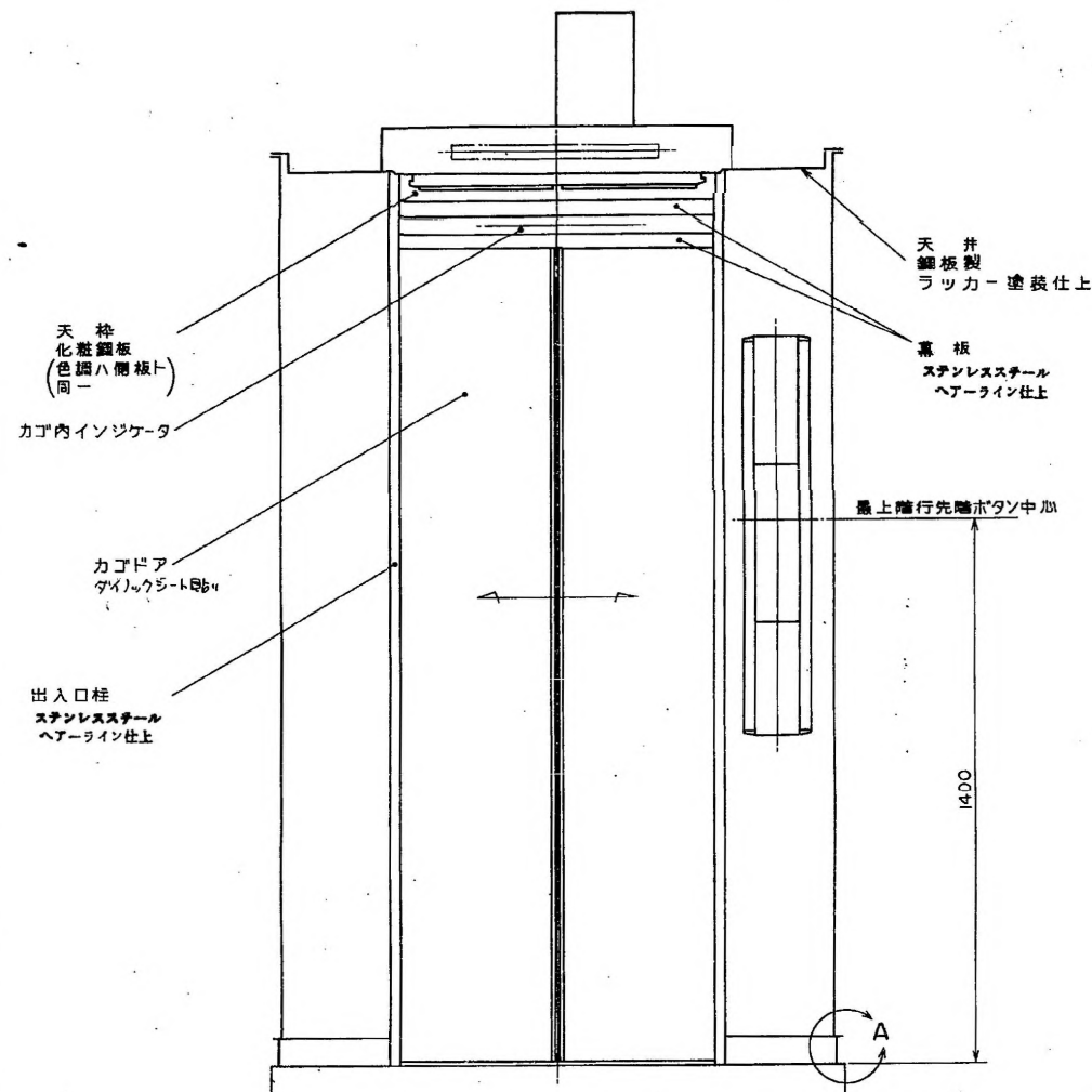
正面図
