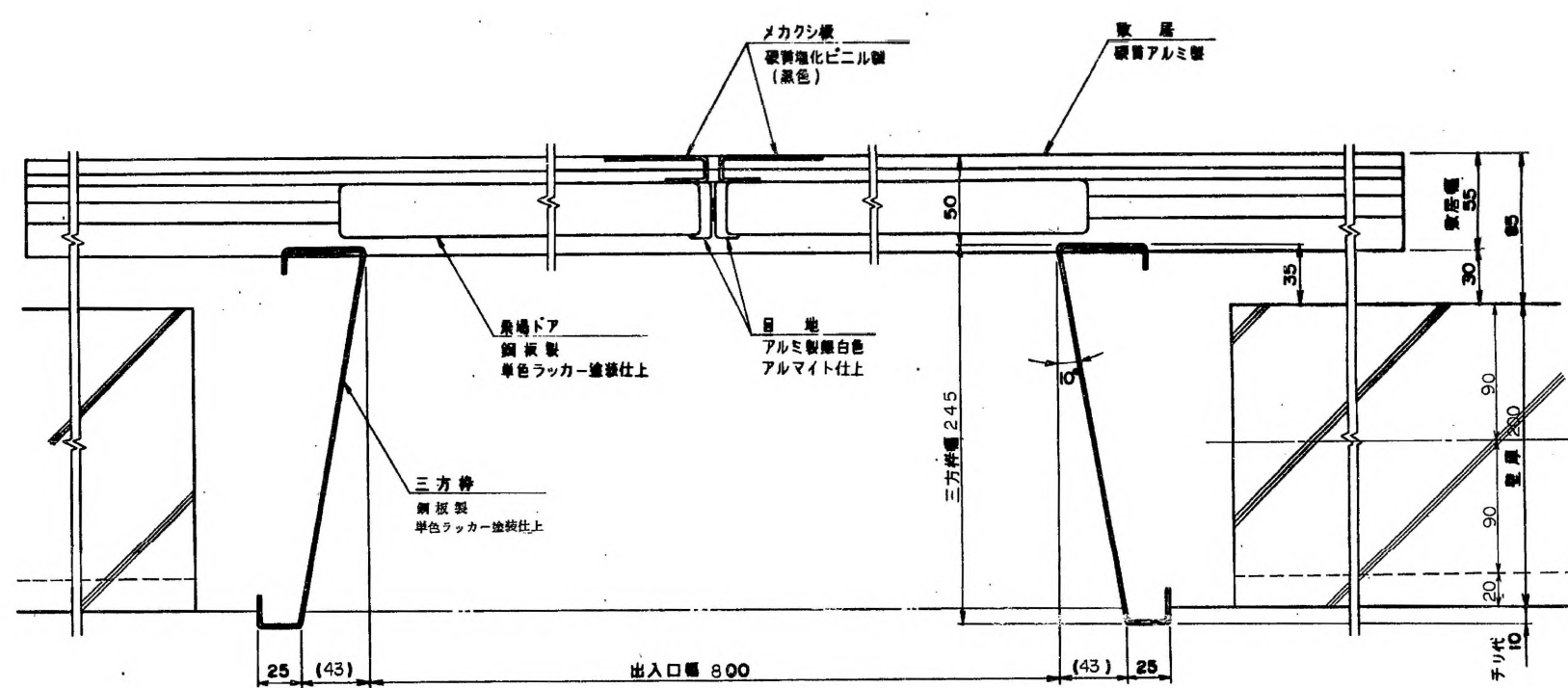
平面図 (1/2)
