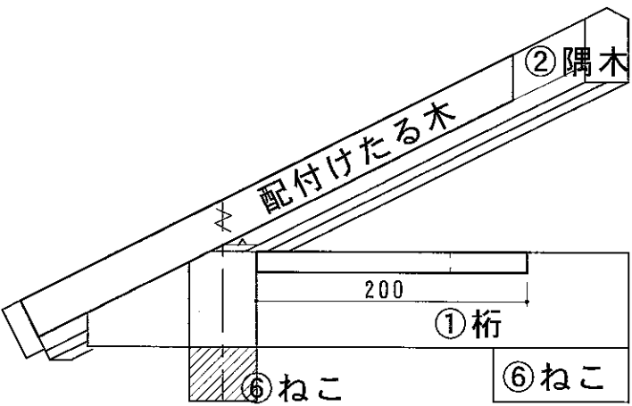
右側面図
