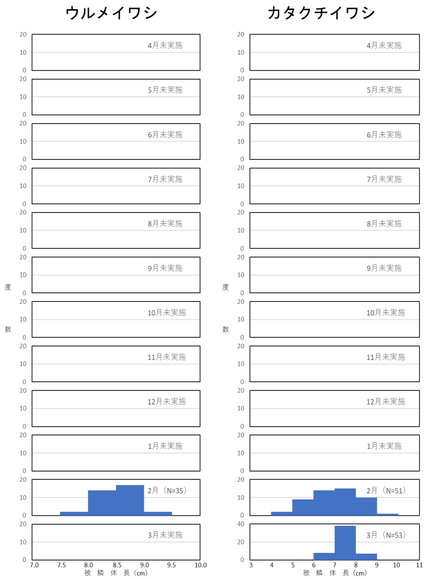
図5 穴喰漁協で漁獲されたいわし類の被鱗体長組成
