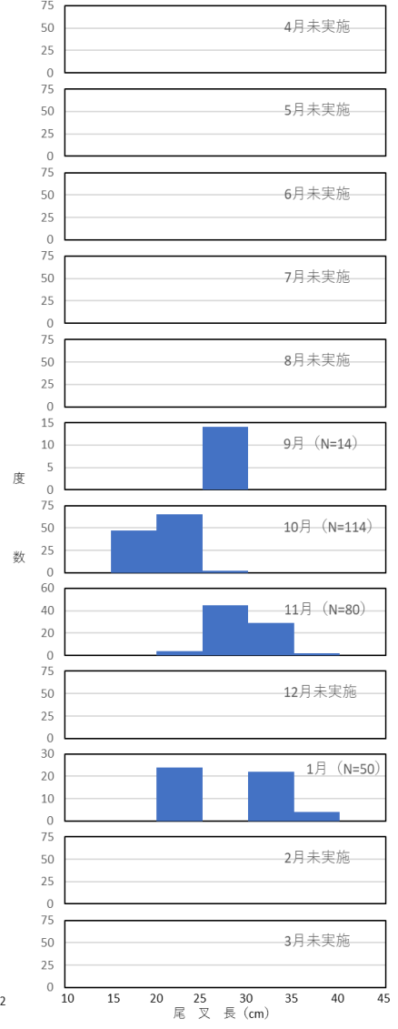
図4 さば類の尾又長組成
