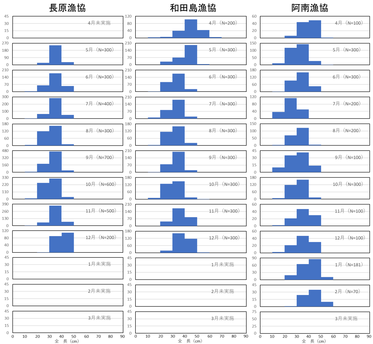
図1 各漁協で漁獲されたカタクチワシラスの全長組成
