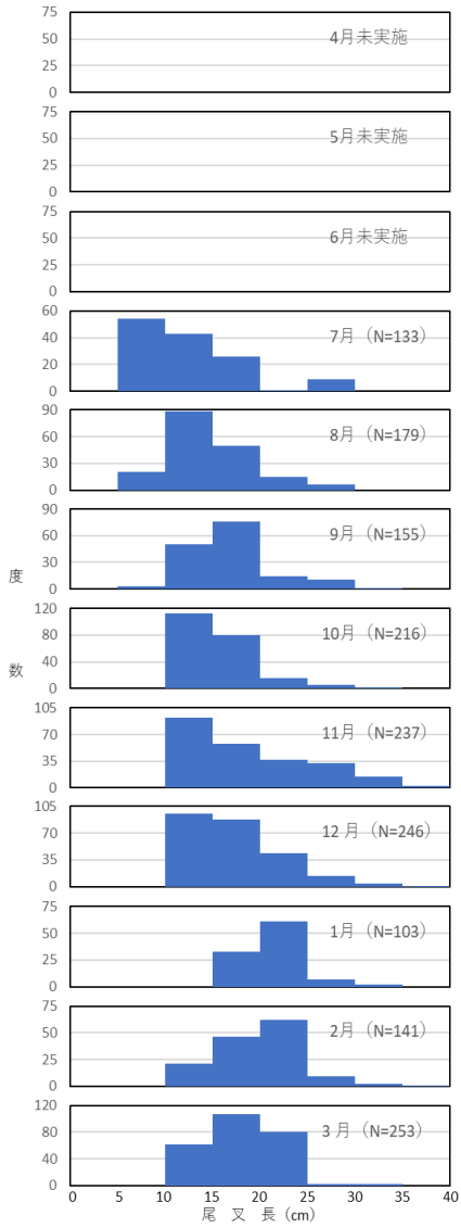
図3 各漁協で漁獲されたマアジの尾又長組成
