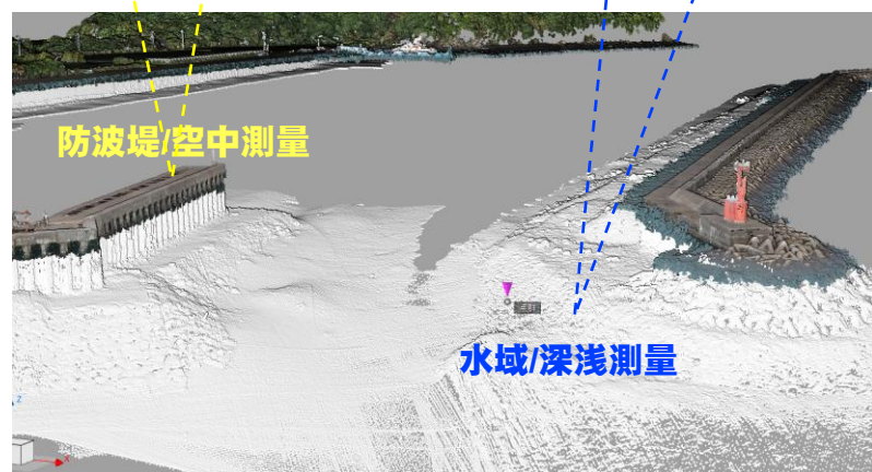
UAV(ドローン)を活用した 沖合施設(離岸堤)の点検
