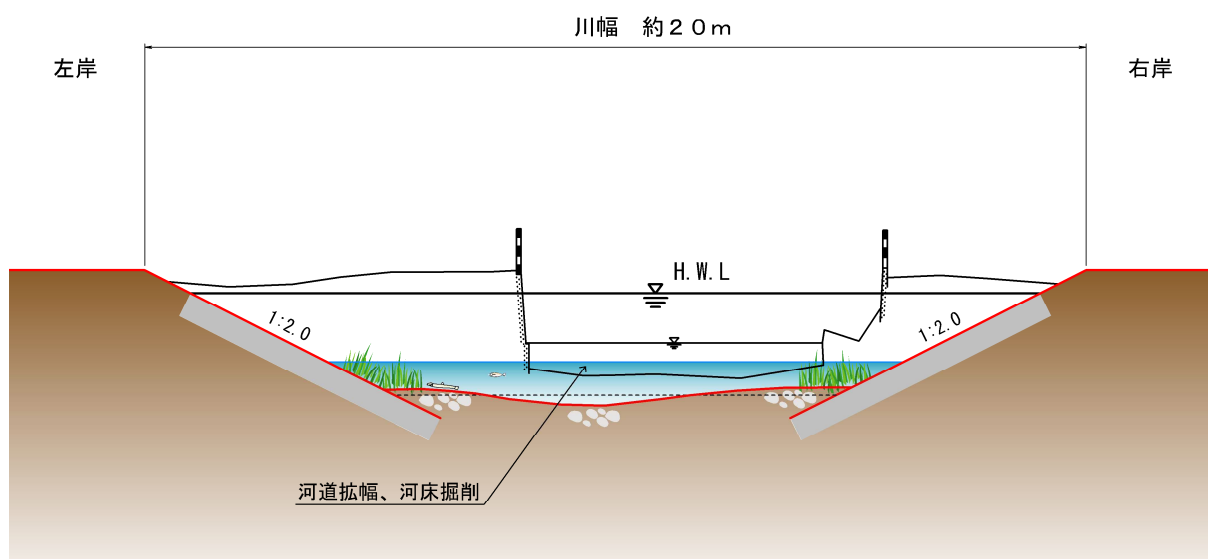
図 4-2 三谷川横断面
