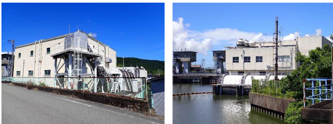
写真 4-1 水位観測施設
