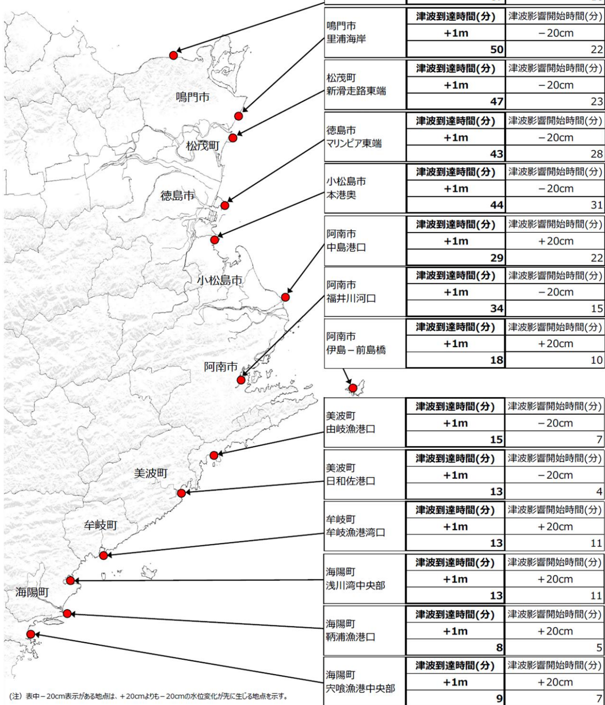
図 2-1-6-1 : 南海トラフ巨大地震による津波到達時間・津波影響開始時間
