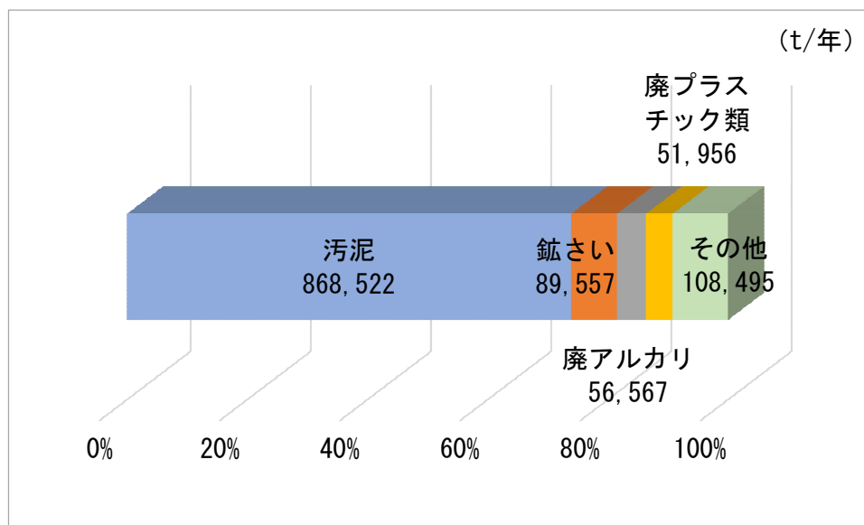
図 23 製造業の種類別排出量（令和5年度）
