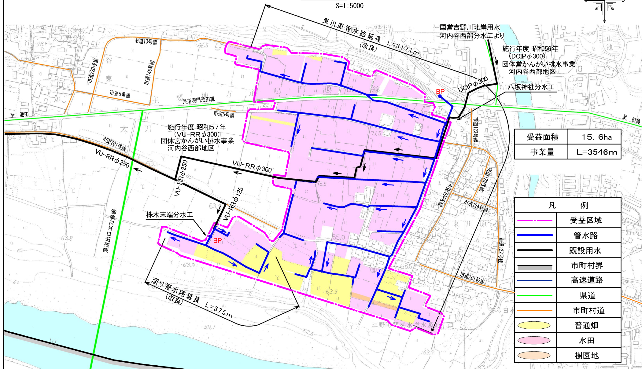
計画平面図
