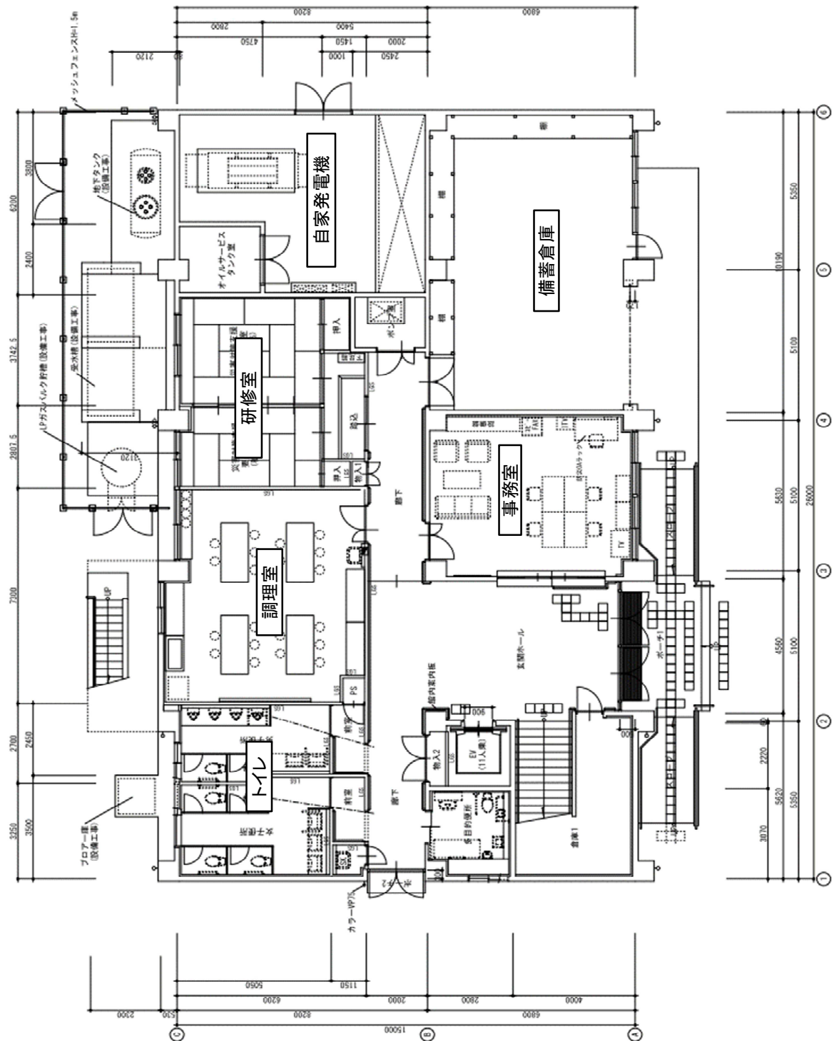
西部防災館(本館) 1階平面図
