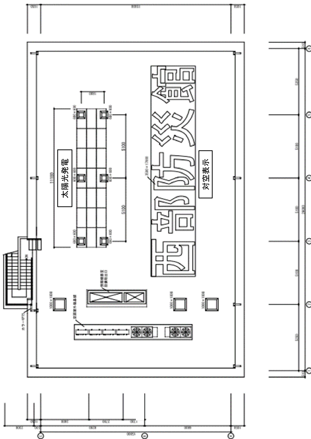
西部防災館(本館) R階平面図
