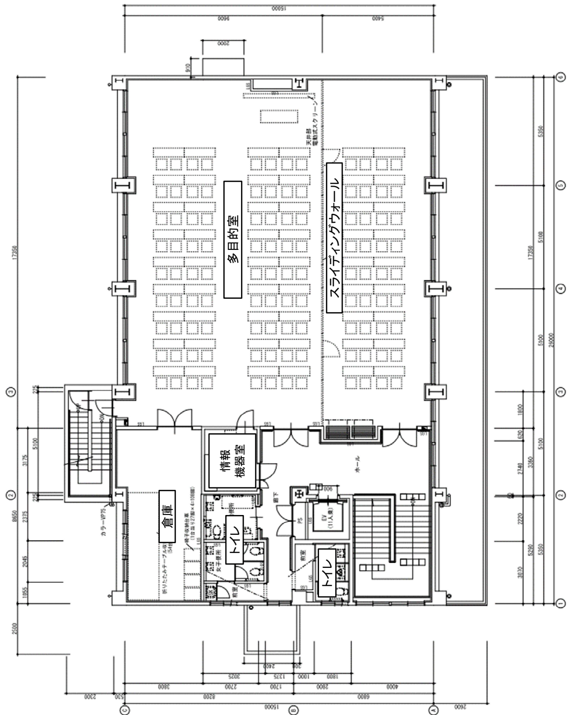
西部防災館(本館) 2階平面図
