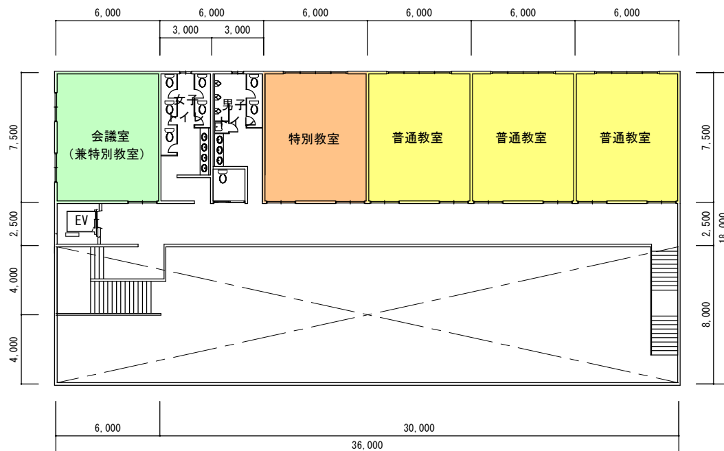
2 階平面図
