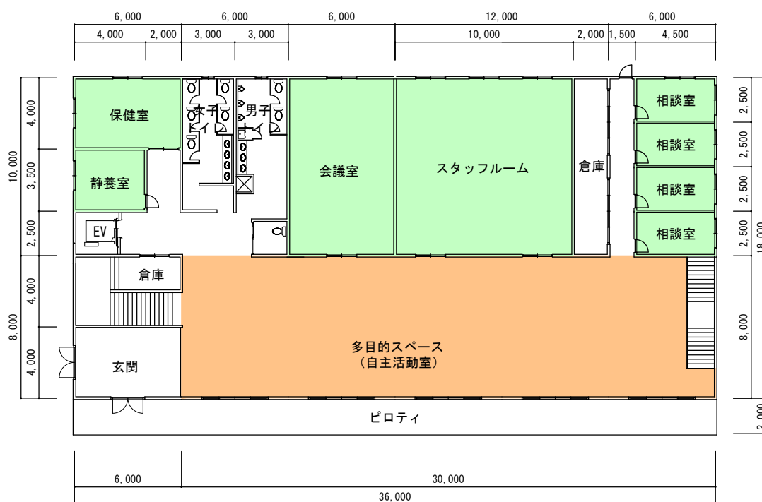
1 階平面図
