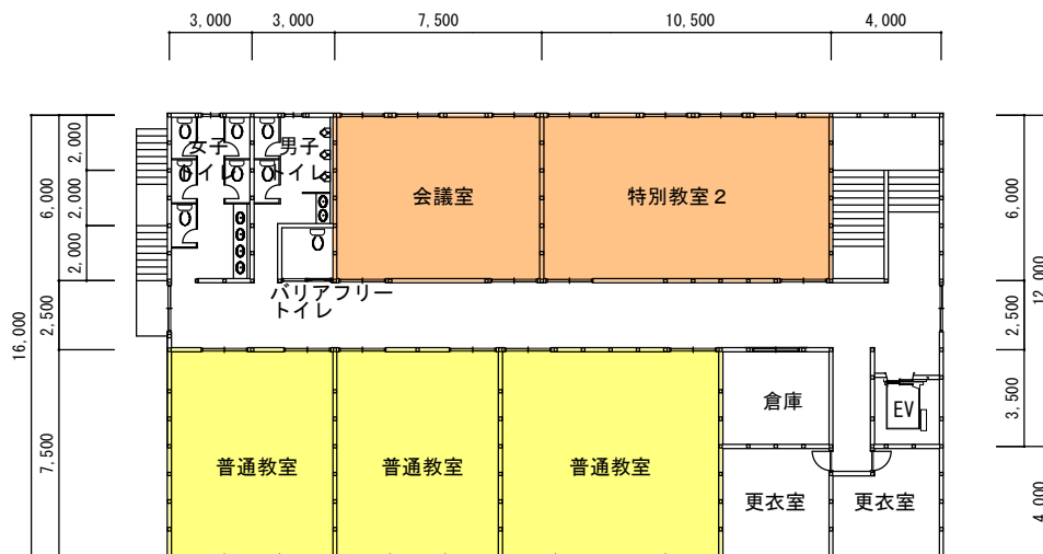
2 階平面図
