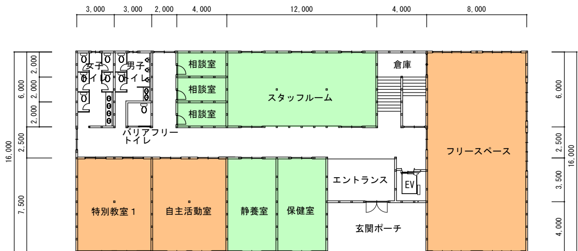
1 階平面図
