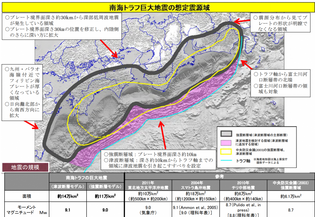
図-5 「南海トラフの巨大地震モデル検討会」公表 想定震源域
