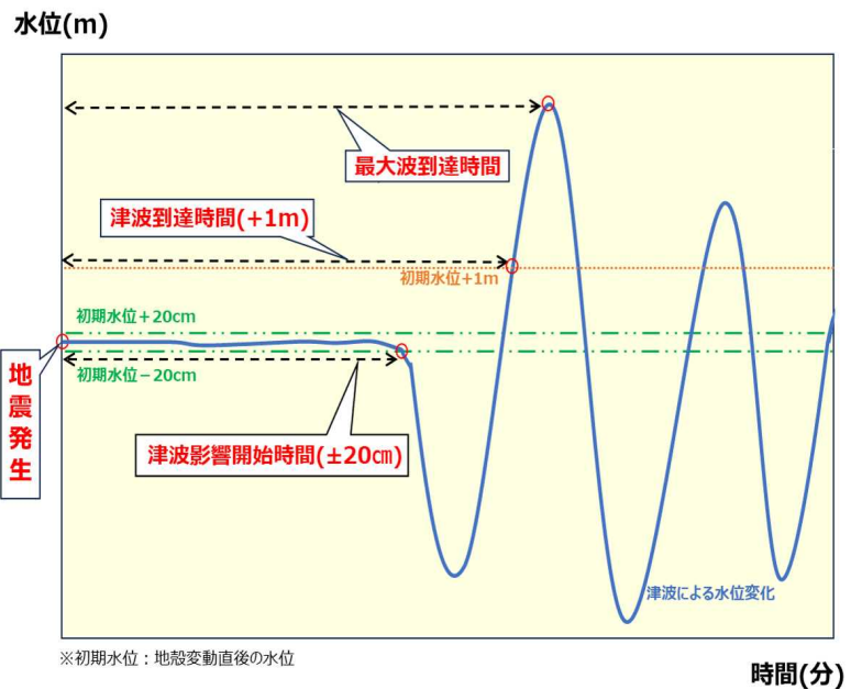
図－4 津波到達時間の計測方法
