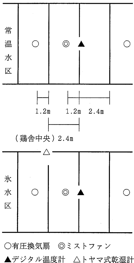
図4. 試験2の設定
