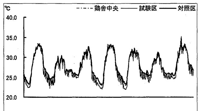
図3. 鶏舎気温の変化
