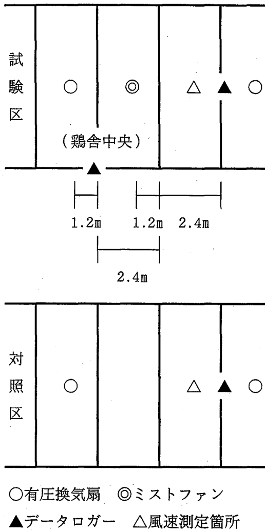
図1. 試験1の設定
