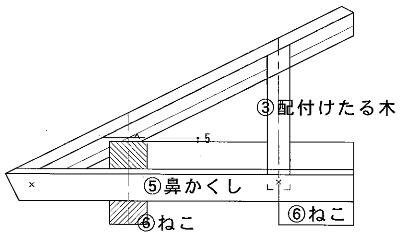
正 面 図
