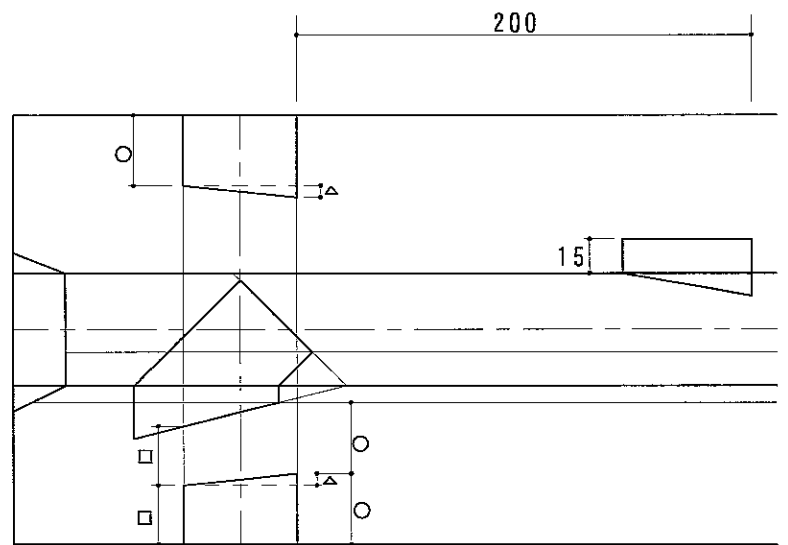
桁ねじ組み詳細図
