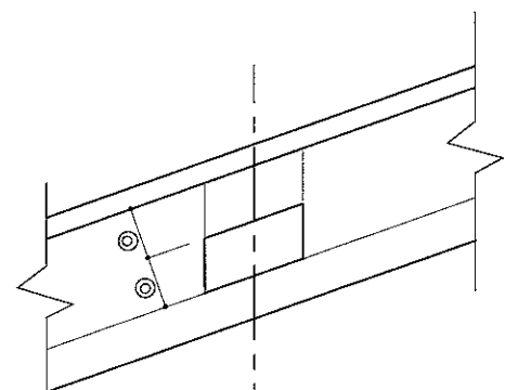
隅木と配付けたる木 取合いほぞ穴詳細図
