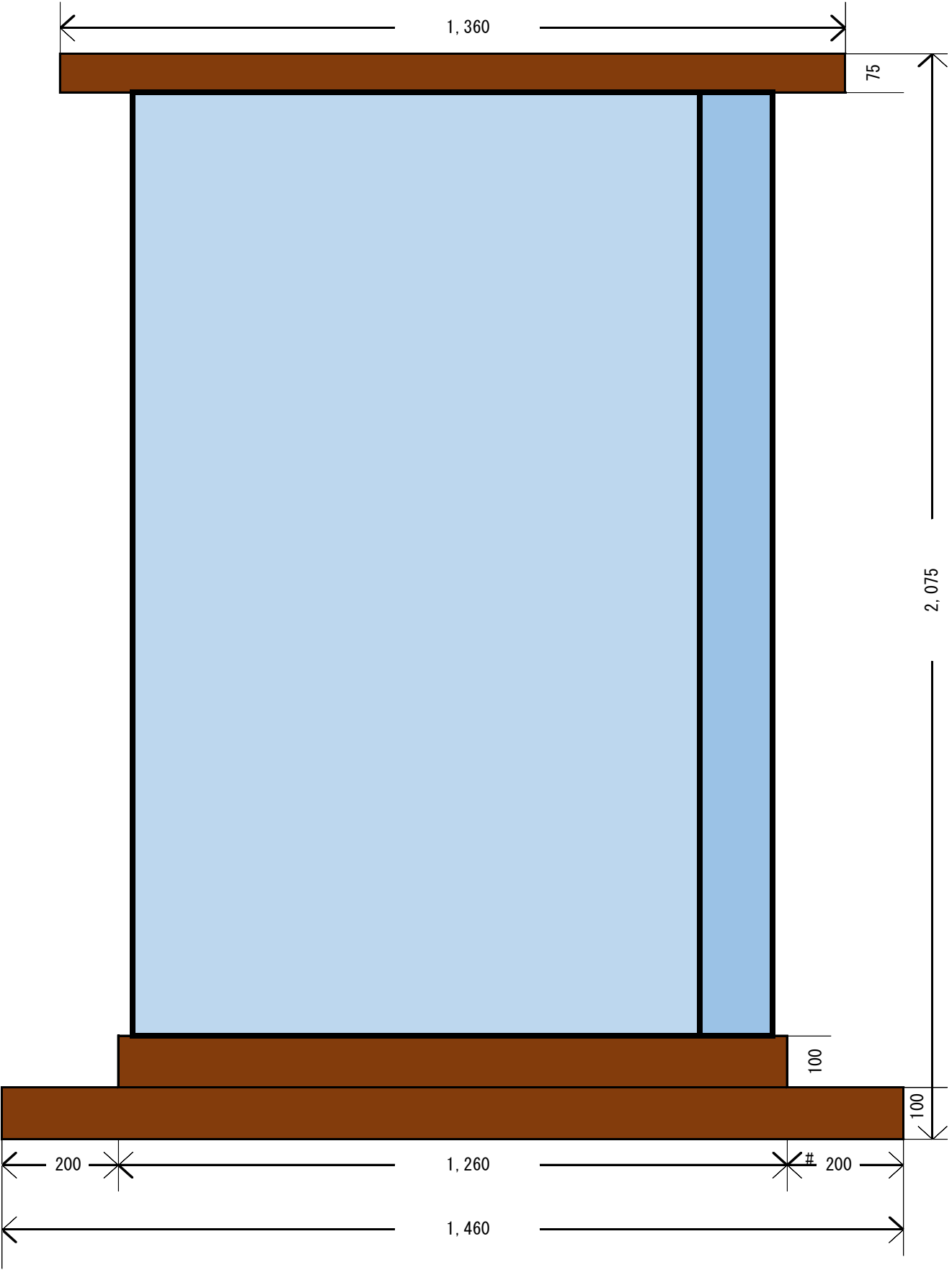
課題図 1 （寸法）
