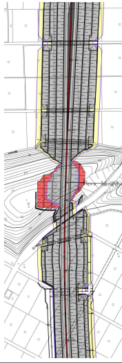
切土法面勾配の変更 (決定区域の増)
