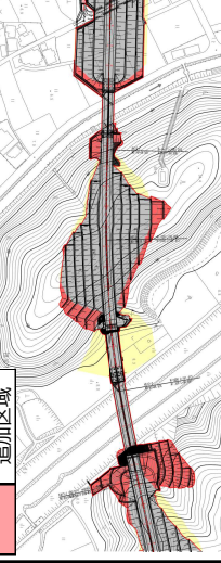
橋台位置見直しに伴う構造変更 (決定区域の増減)
