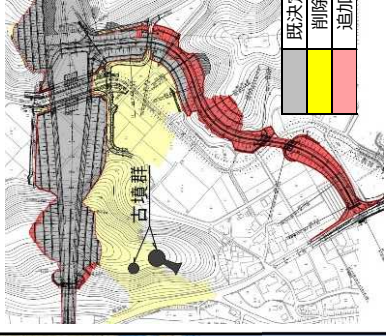
埋蔵文化財保護に伴うルートの変更
