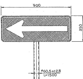
誘導標2型
