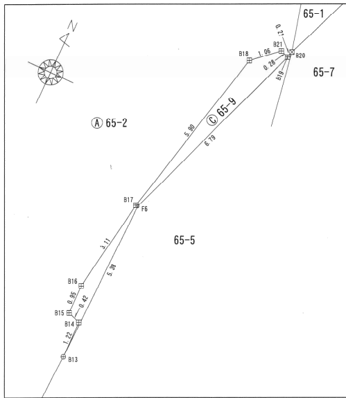
拡大図1 縮尺:1/100
