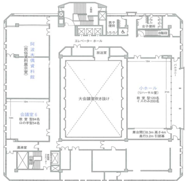
5階
